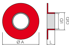
TYPENREIHE SFR MIT RUNDFLANSCH
