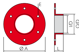
TYPENREIHE SFRB MIT RUNDFLANSCH UND VORGEBOHRTEN LÖCHERN
